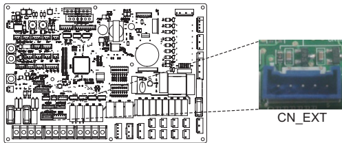
Vnitřní DPS
