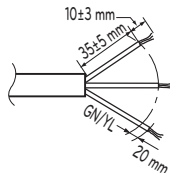
Pro 1 fázi
