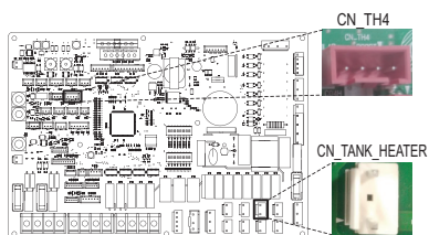
Vnitřní DPS
