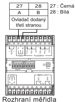
Rozhraní měřidla
