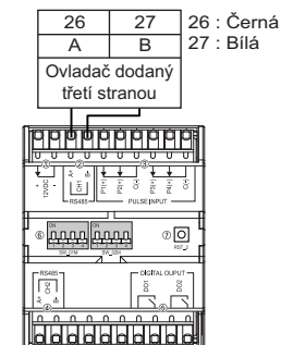
Rozhraní měřidla
